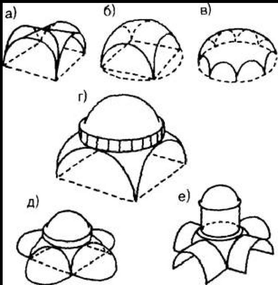
СХЕМА КОНСТРУКТИВНОГО РАЗВИТИЯ ВИЗАНТИЙСКОГО «КУПОЛА НА ПАРУСАХ»
