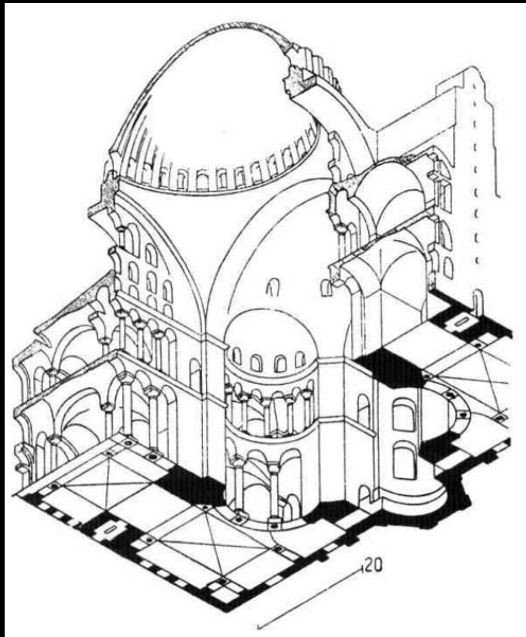
АКСОНОМЕТРИЧЕСКАЯ СХЕМА ХРАМА СВЯТОЙ СОФИИ В КОНСТАНТИНОПОЛЕ
